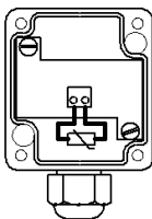
2-Leiteranschluss
