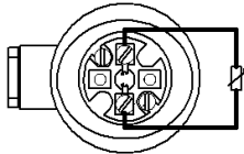
2-Leiteranschluss
