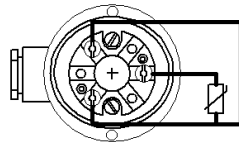
3-Leiteranschluss
