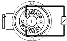
2-Leiteranschluss
