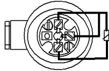
3-Leiteranschluss
