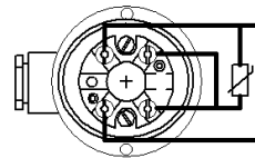
4-Leiteranschluss
